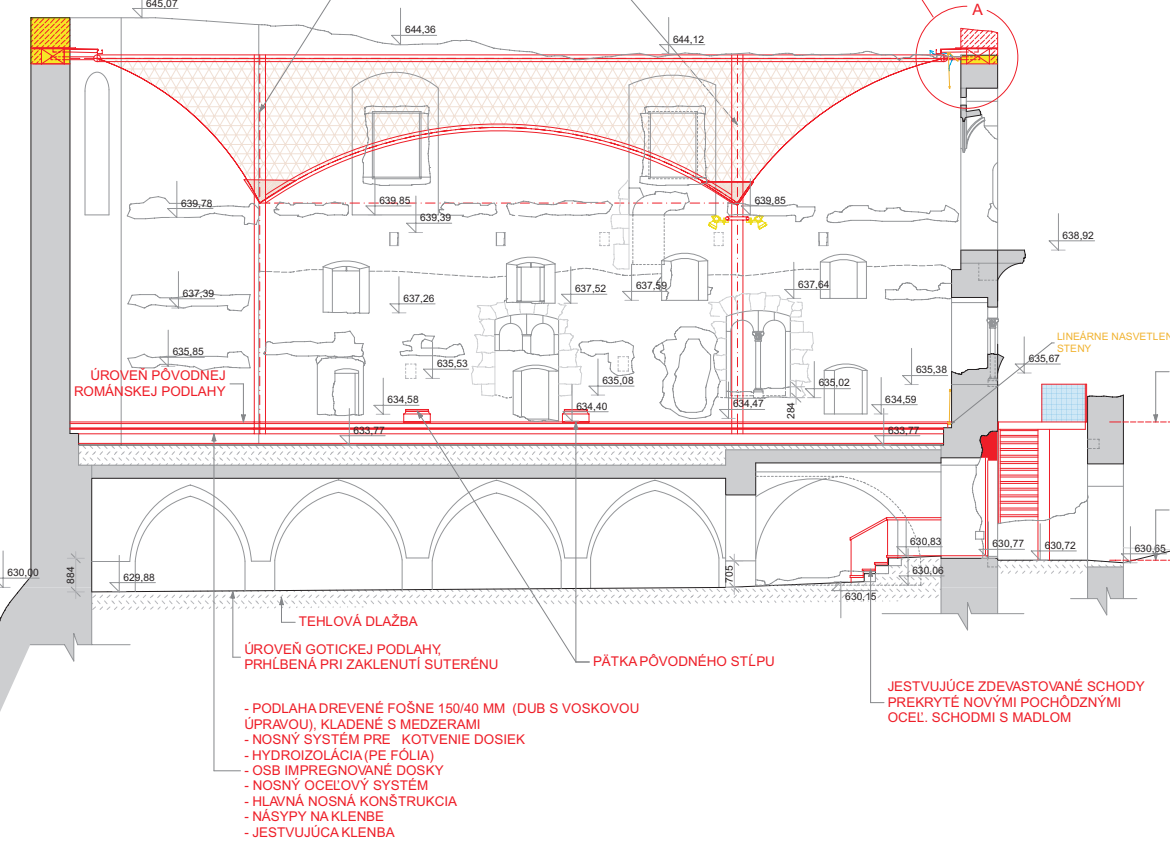
Románsky palác rez B - B
