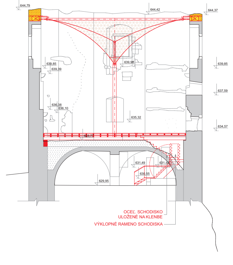
Románsky palác rez D - D
