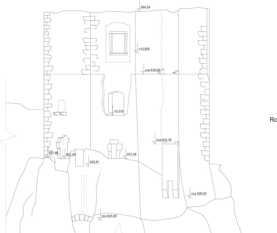
Románsky palác pohľad juhovýchodný 2
