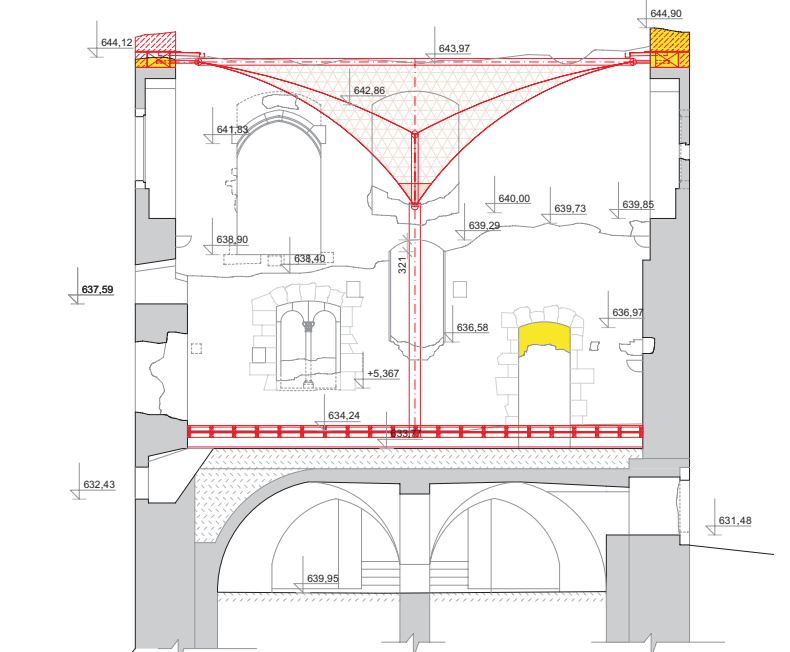
Románsky palác rez C - C
